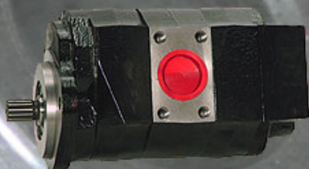
JCB EJE 15 ESTRIAS 1"
